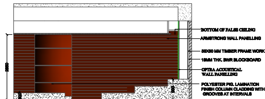
WALL ELEVATION E
